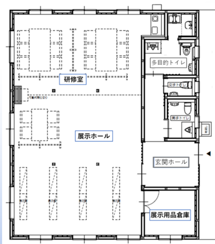
施設平面図
